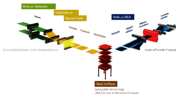
Abb. 2 Der H2GO-Verbund Stack2P (Stack to Piece) untersucht, welche Maschinen, Anlagen und Prozesse benötigt werden, um Brennstoffzellensysteme automatisiert montieren und am Ende ihres Produktlebens zerstörungsfrei wieder demontieren zu können. Projektpartner sind die Fraunhofer-Institute IST, IWU, IKTS und IFAM © Fraunhofer IWU www.iwu.fraunhofer.de
